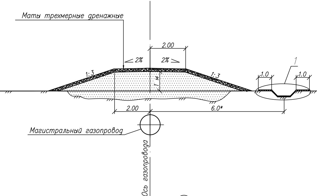
Схема поперечного профиля
